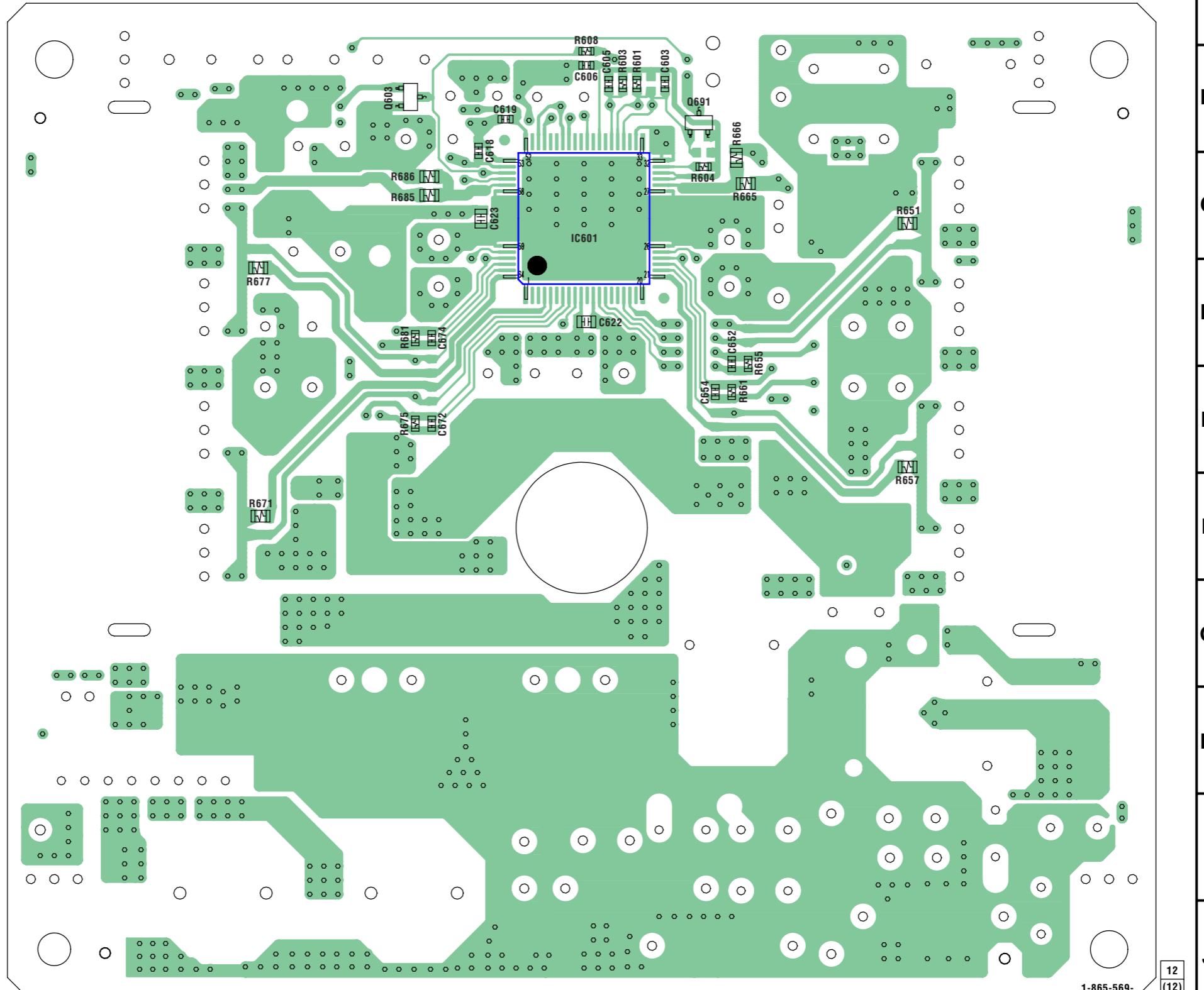
【AMP BOARD】(SIDE A)
